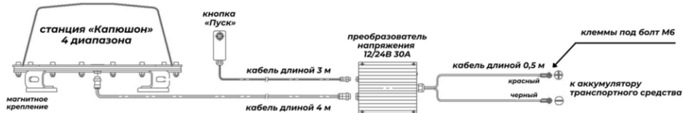
Схема установки станции Капюшон на грузовой автомобиль с напряжением бортовой сети 24В
